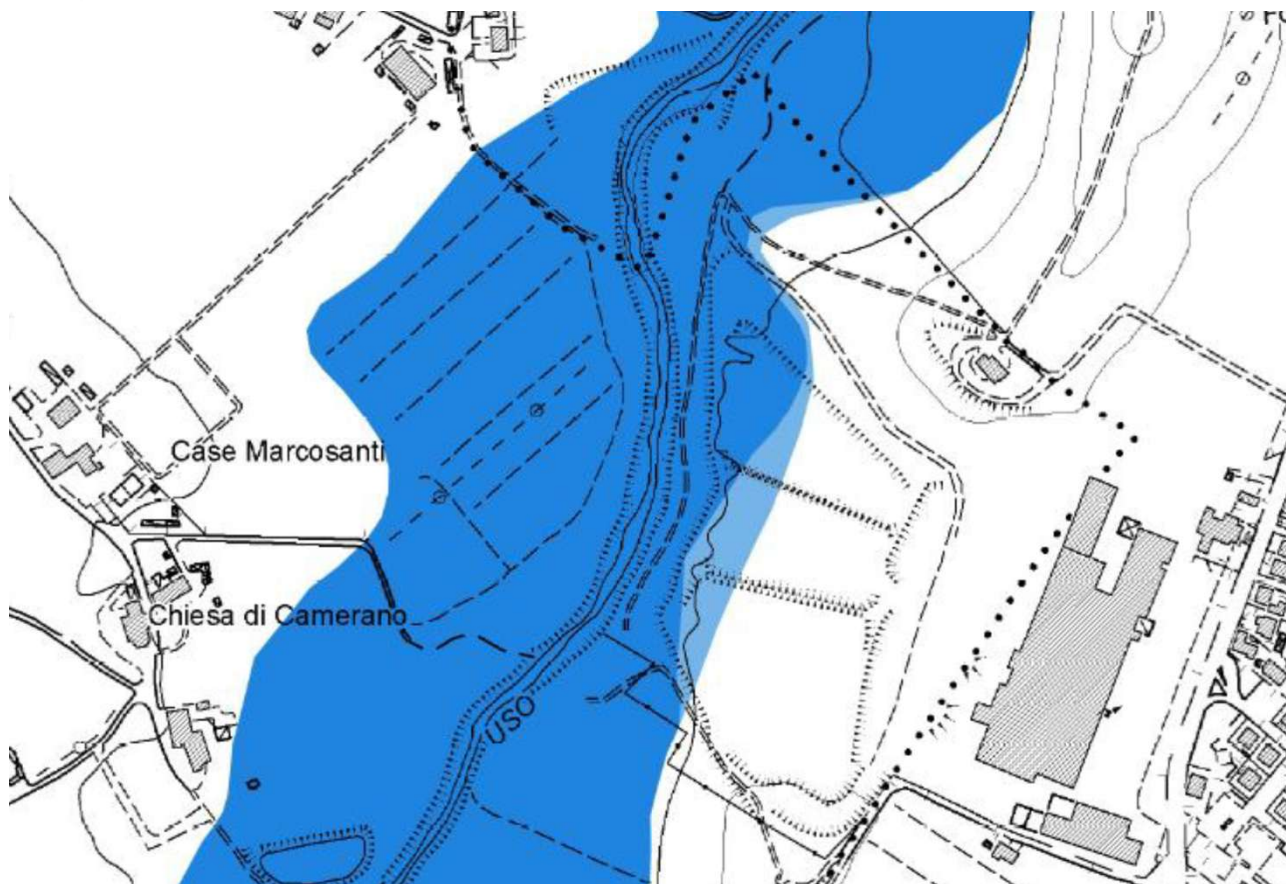
Fig. 9 – stralcio della mappa PGRA_USO_2 relativa al PGRA 2027. Il sito Ripa Bianca viene lambito da un'area P2 (azzurro chiaro) e da un'area P3 (azzurro scuro).
