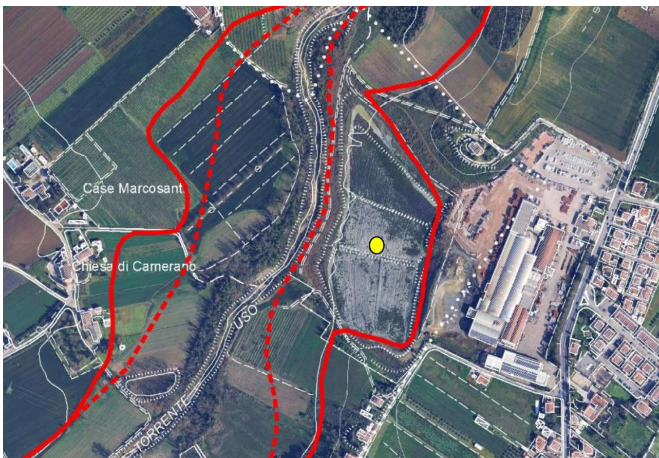
Fig. 8 stralcio della tavola PAI_FASCE_FLUVIALI_USO2. Il sito di cava Ripa Bianca (punto giallo) è ricompreso in una fascia B in destra idrografica.
